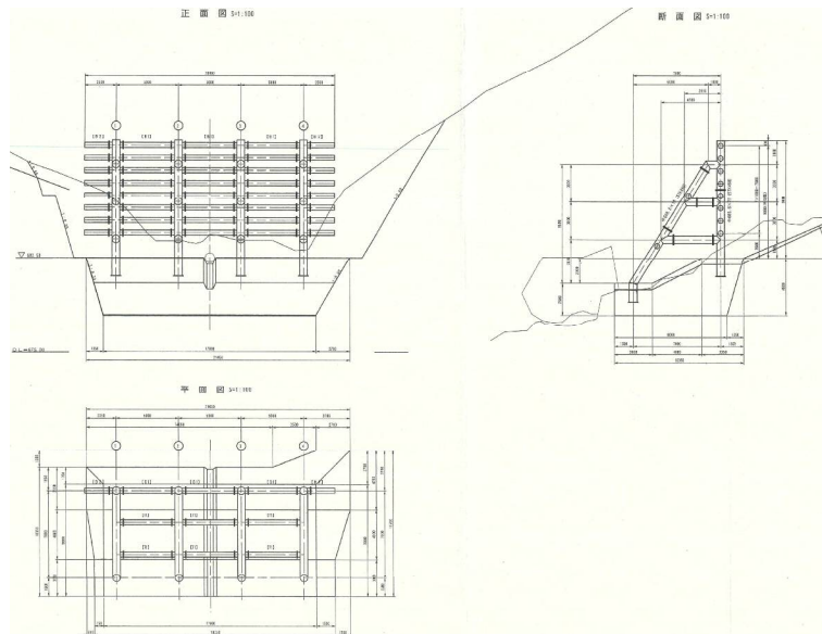
雪崩減勢柵構造一般図 3)
