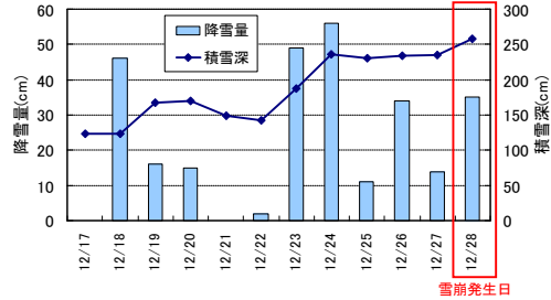
雪崩発生日までの降雪量と積雪深 1)
