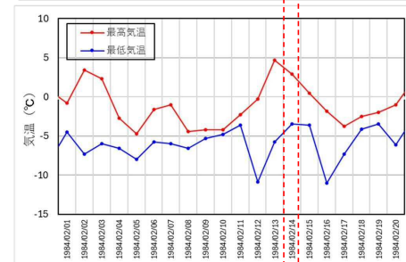
気象データ 3) を加工
