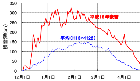
積雪深の傾向 2)
